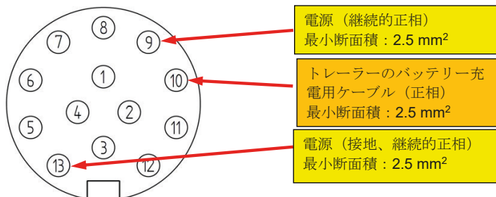
ISO11446:2004 対応の 13 ピンプラグの配線
