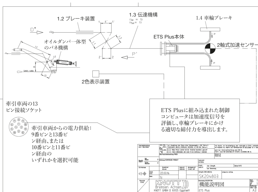
後付けETSブレーキ装置の全体
