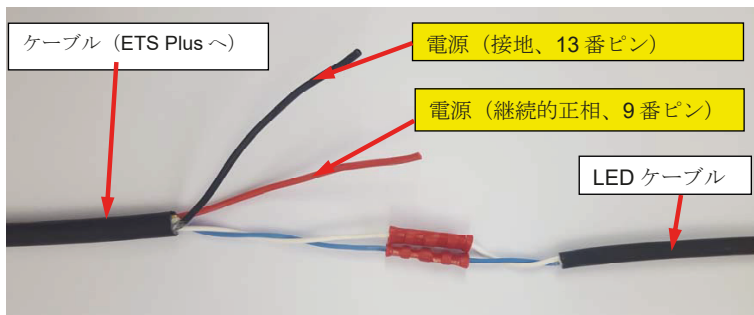
図： ETS Plus の配線（キャラバン使用者用の電気的機能無し）
