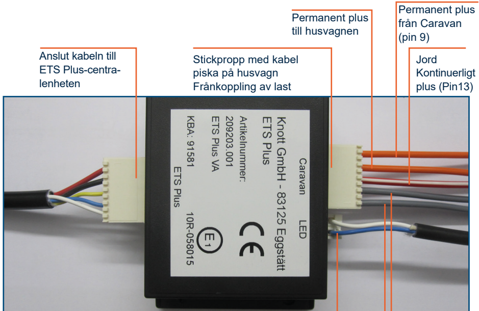
ETS Plus-kablage med Husvagnsavstängning
