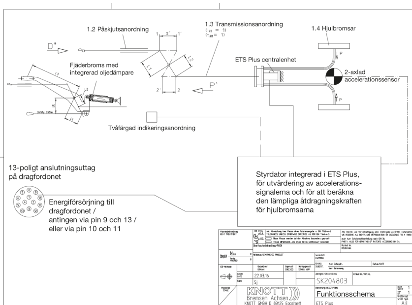
Schema över ETS-bromsanläggningen som installeras i efterhand
