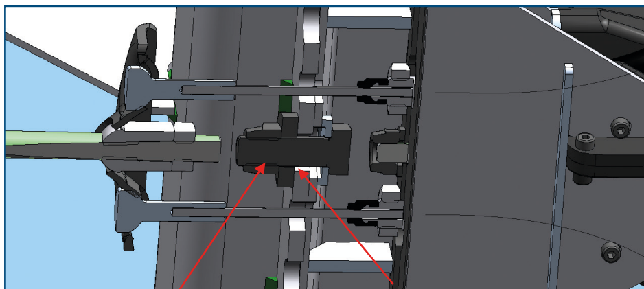
Contratuercas M12 Par de apriete 80 +10Nm
