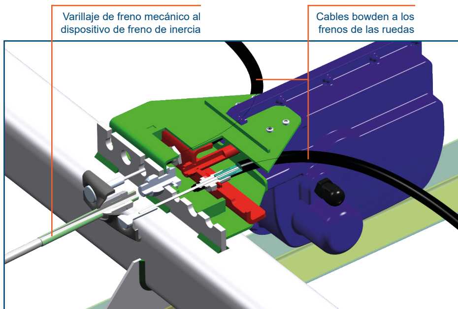
Vista detallada de la unidad central del ETS Plus en el contrasorte de cables bowden del eje
