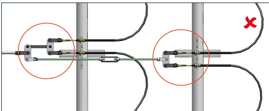
Caso III: Tandem com balanças de compensação por eixo
