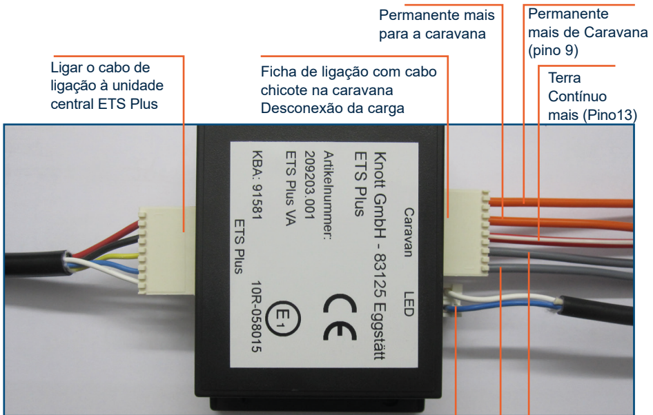
Cablagem ETS Plus com Desligamento do consumidor para caravanas
