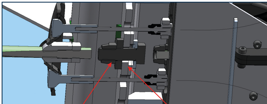
Contra-porca M12 Binário de aperto 80 +10 Nm
