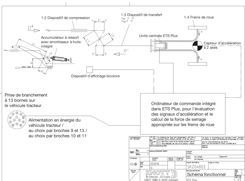
Figure: Schéma du système de freinage ETS pour un équipement ultérieur
