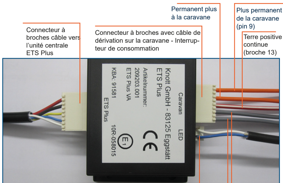
Câblage ETS Plus avec caravane système de désactivation des consommateurs
