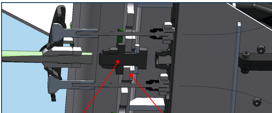
Dado di bloccaggio M12 Piastrina Coppia di serraggio di 80 +10 Nm
