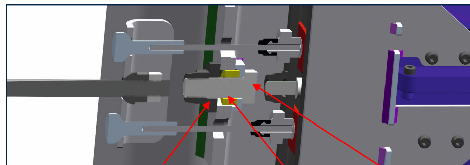
Dado di bloccaggio M12 Piastrina Boccola di centraggio Coppia di serraggio di 80 +10 Nm
