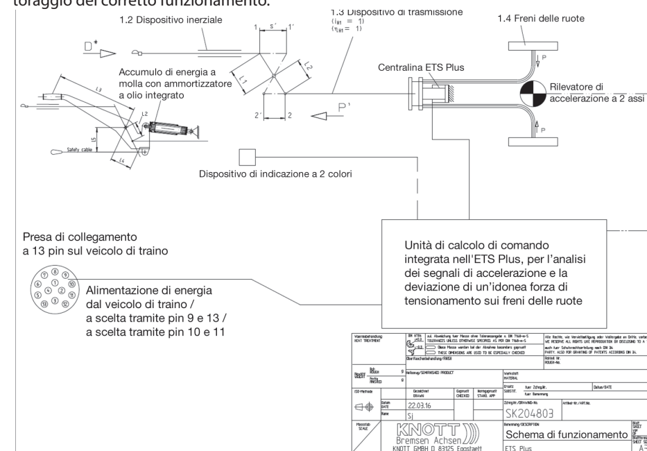
Immagine: Schema dell'impianto frenante ETS per retrofit
