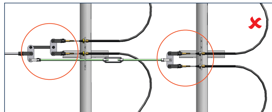
Caso III: Tandem con stabilizzatori per ogni assale
