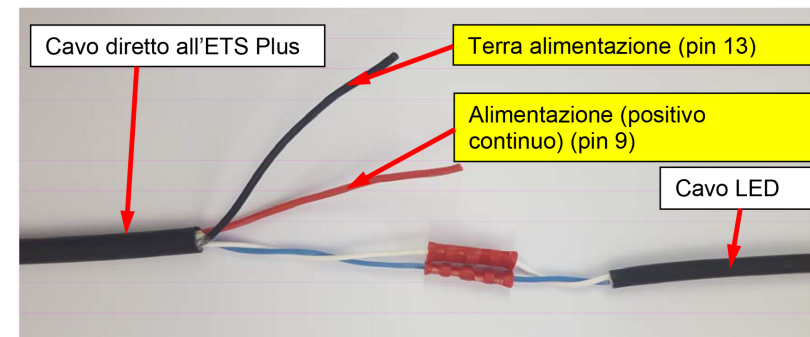
Immagine: Cablaggio dell'ETS Plus senza dispositivo di messa in sicurezza elettrica delle utenze sulla roulotte
