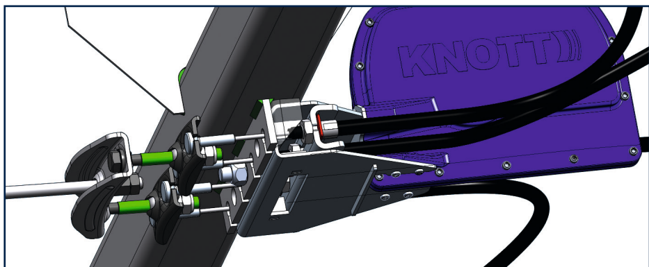
Immagine: Tirante del freno completamente premontato con centralina ETS Plus
